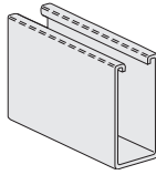
1501-1542 1 5 / 8 " X 3 1 / 4 " X 12 Ga.
