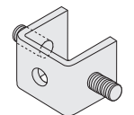
STUD RING CONNECTOR 5541 1 Stud 5542 2 Stud 5543 2 Stud (Shown)
